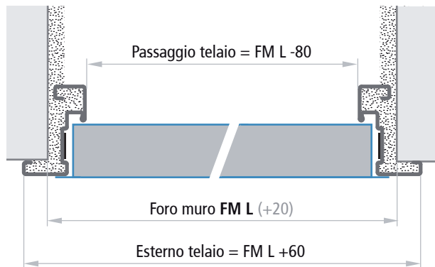
Porta ad un'anta Sezione orizzontale
